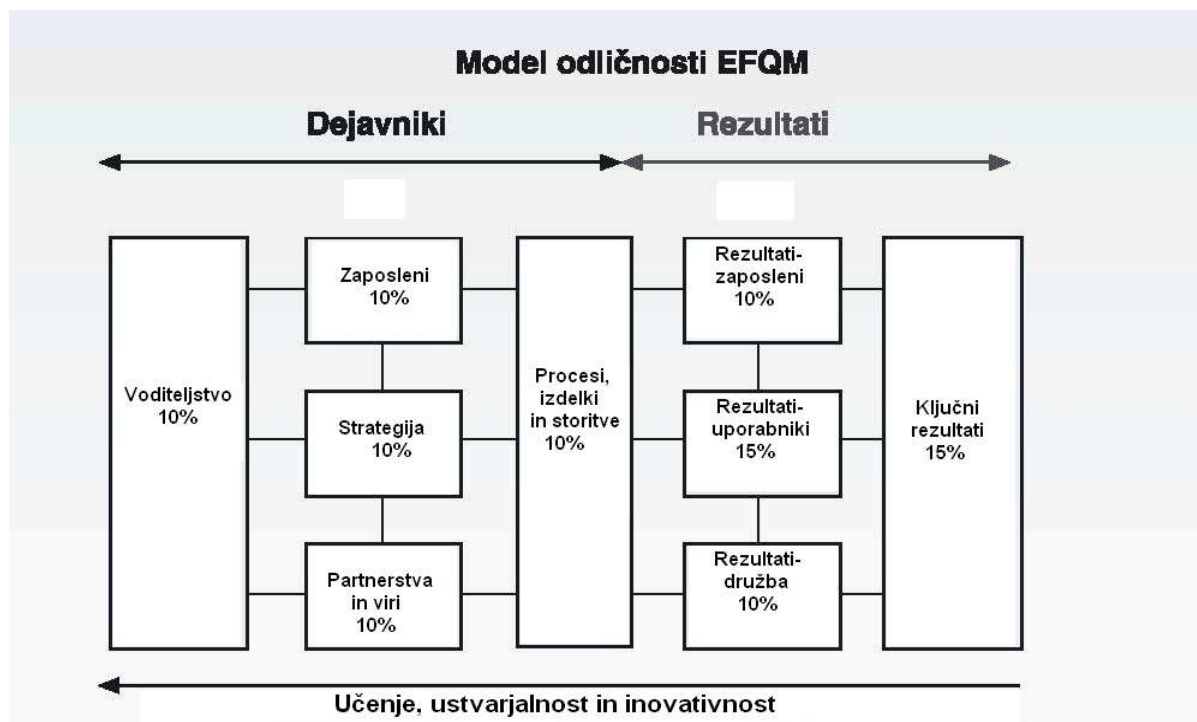
Slika 8: Model EFQM 2010
