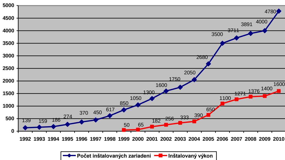
Graf 2 - Počet inštalovaných bioplynových elektrární a celkový inštalovaný výkon v MW v Spolkovej republike Nemecko od roku 1992 5
