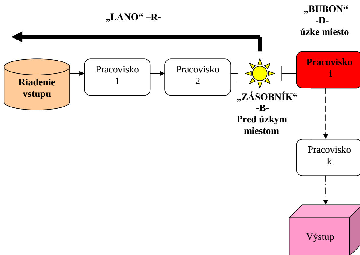
Obr. 3 Štruktúra výrobného procesu DBR
