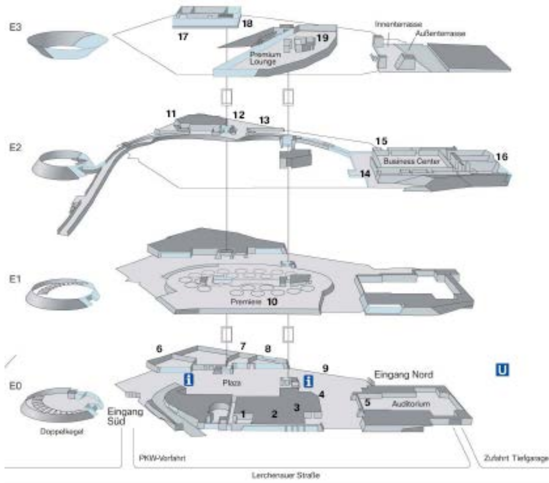
Abbildung 7: Layout und Ebenen der BMW Welt 47
