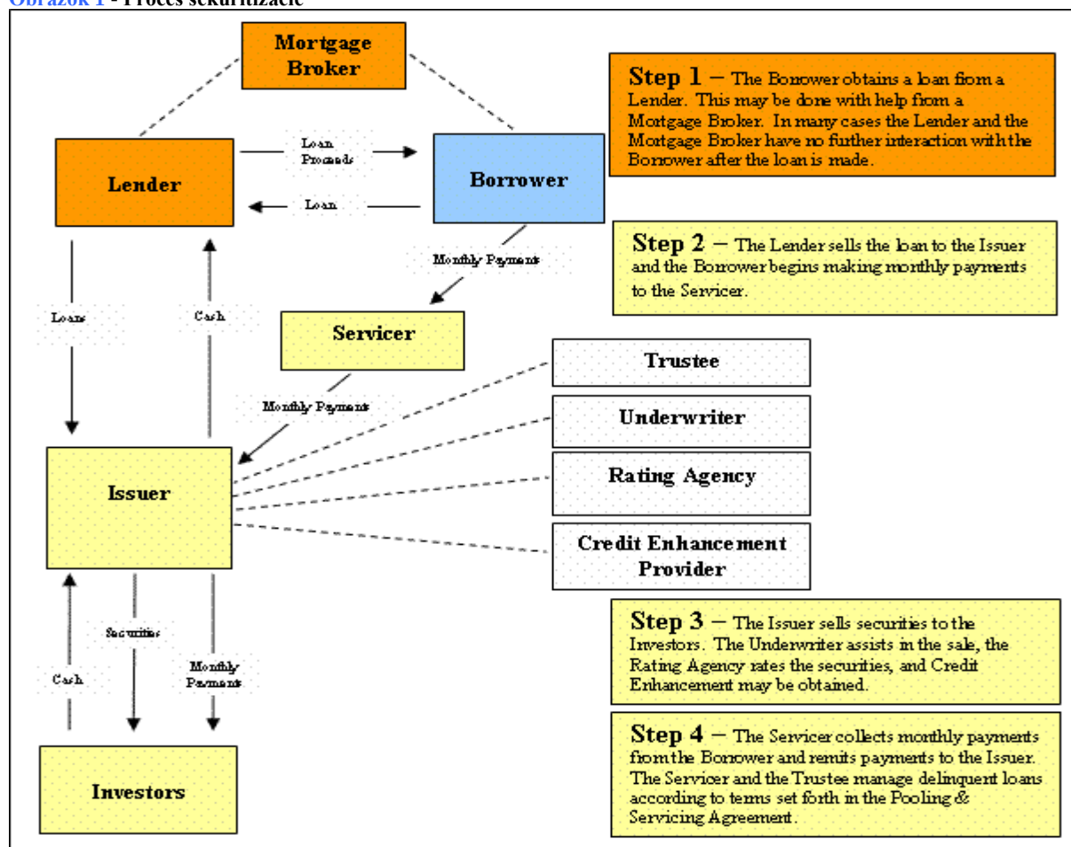
Obrázok 1 - Proces sekuritizácie
