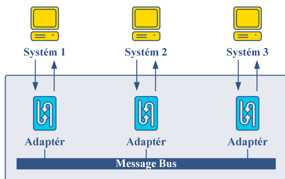
Obrázek 11 Message Bus
