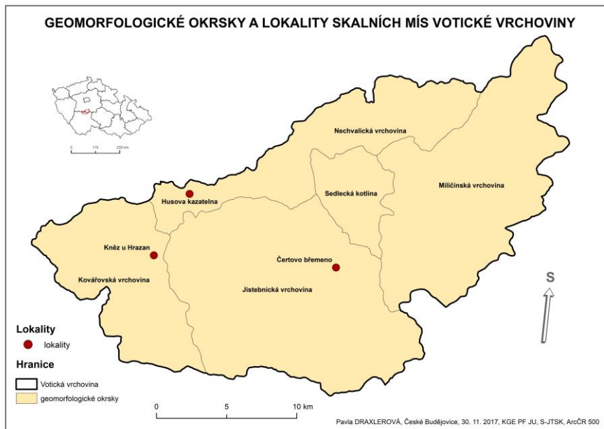
Mapa 1: Geomorfologické okrsky a lokality skalních mís Votické vrchoviny
