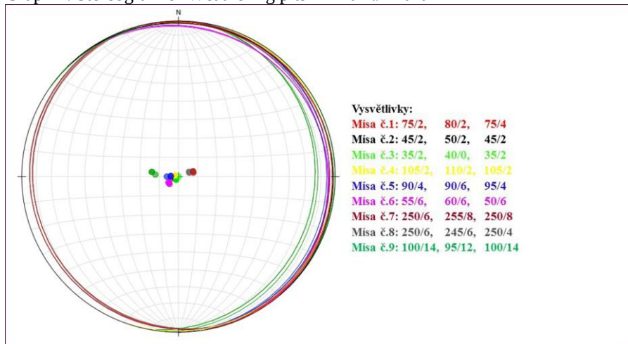
Graf 2: Stereogram skalních mís – Kněž u Hrazan
