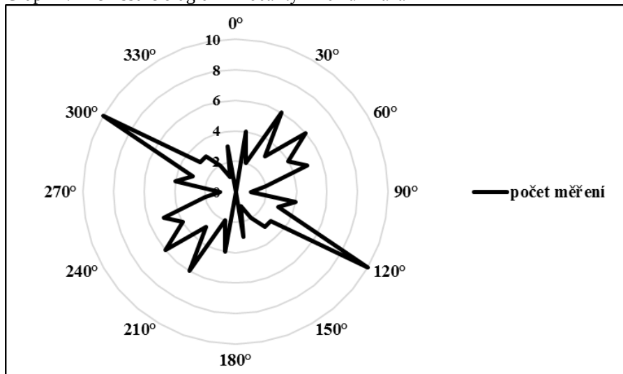
Graf 1: Puklinový diagram – lokalita Kněž u Hrazan
