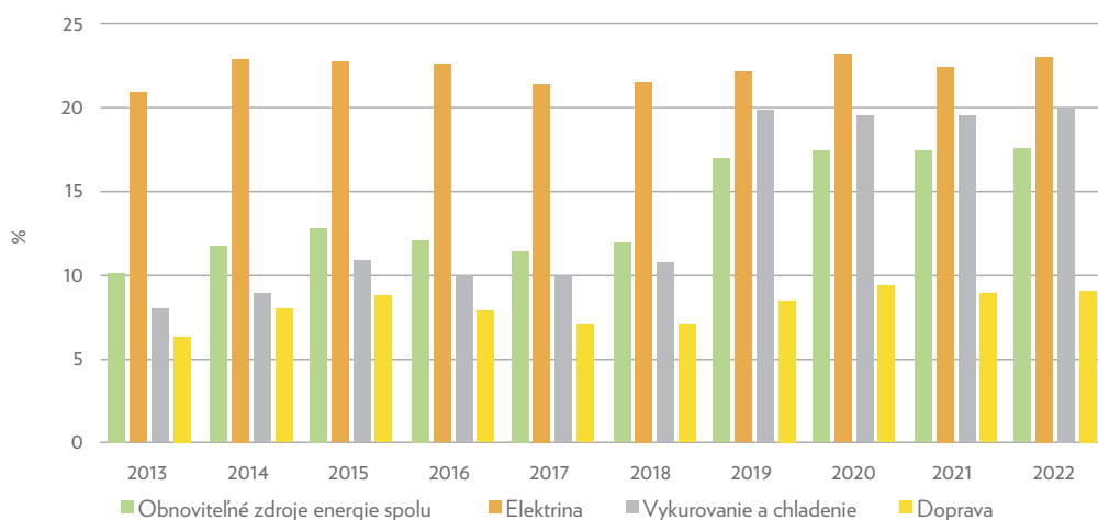
Graf 43 Podiel energie z obnoviteľných zdrojov podľa sektorov na Slovensku (v %)
