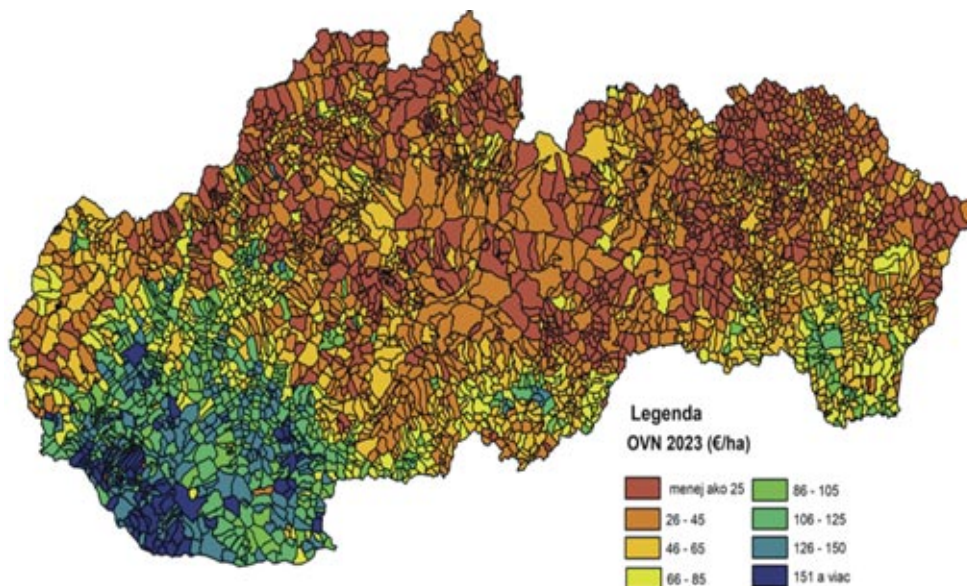
Mapa 7 Priemerná obvyklá výška nájomného v SR v roku 2023 za poľnohospodársku pôdu (€/ha)
