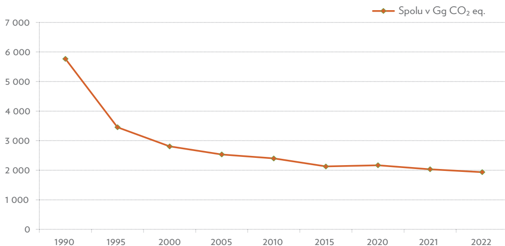
Graf 46 Vývoj emisií skleníkových plynov z poľnohospodárstva v rokoch 1990 – 2022
