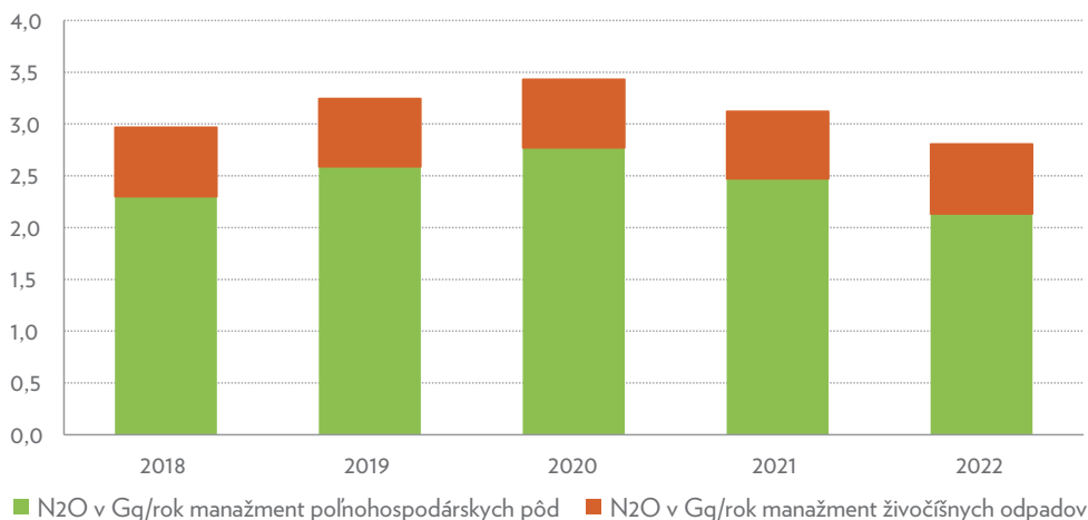
Graf 47 Vývoj emisií oxidu dusného z manažmentu poľnohospodárskych pôd a manažmentu živočíšnych odpadov v rokoch 2016 – 2022
