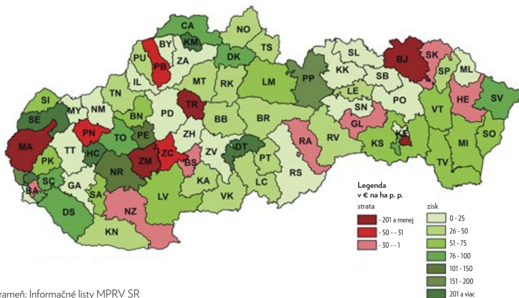
Mapa 4 Výsledok hospodárenia SHR za rok 2023 (v € na ha poľnohospodárskej pôdy)
