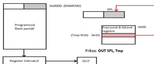
Obr. 7 Schéma realizácie príkazu OUT SPL, Tmp
