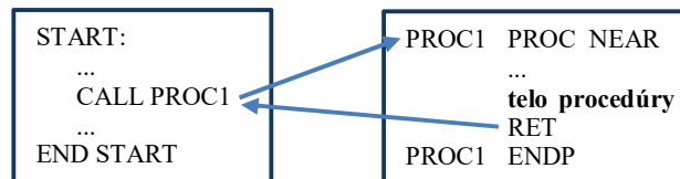
Obr. 3 Schéma činnosti párových inštrukcií CALL – RET
