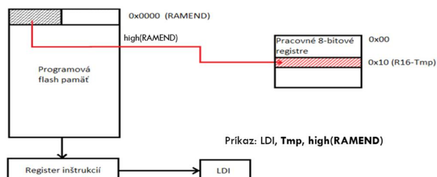
Obr. 8 Schéma realizácie príkazu LDI, Tmp, high(RAMEND)
